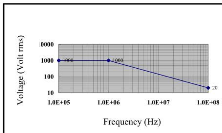
最大绝对输入电压测试曲线图:
