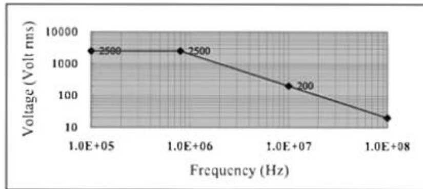
最大绝对输入电压测试曲线图：
