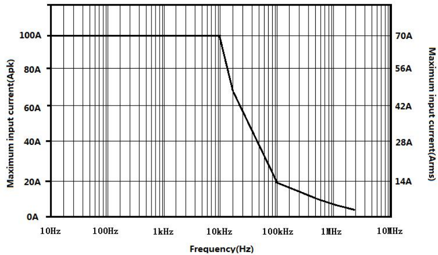
图 3 最大电流 VS 频率特性曲线
